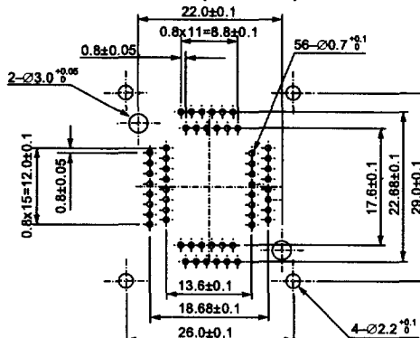
IC51-0564-924 (56 Pins)
