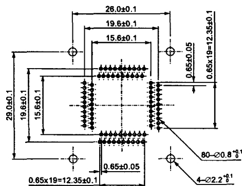
IC51-0804-956-2 (80 Pins)
