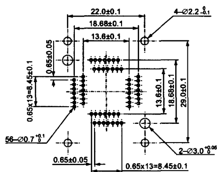
IC51-0564-680 (56 Pins)
