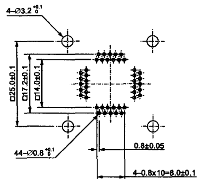
IC51-467-KS11787 (44 Pins)
