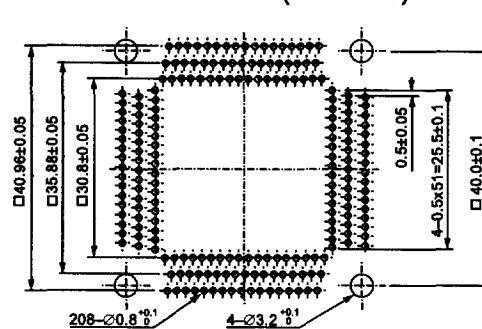
IC51-2084-1509 (208 Pins)
