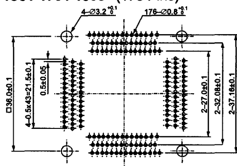
IC51-1764-1505 (176 Pins)
