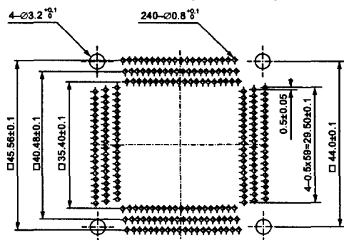
IC51-2404-1655-3 (240 Pins)
