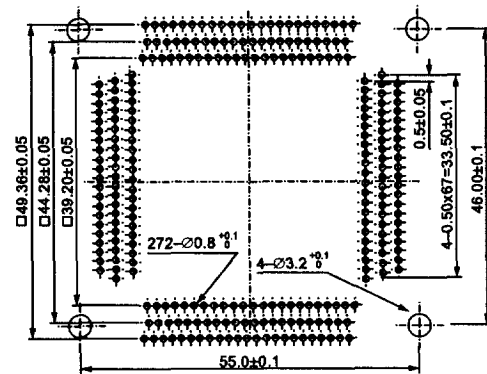
IC51-3044-1471-2 (304 Pins)
