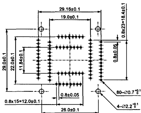
IC51-819-KS12720 (80 Pins)
