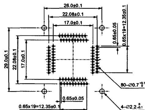
IC51-0804-795 (80 Pins)
