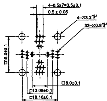
IC51-0324-805 (32 Pins)
