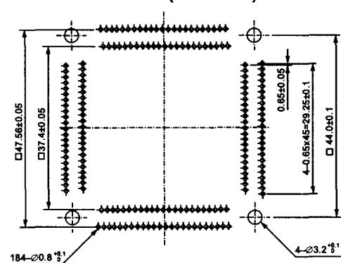
IC51-1844-1541 (184 Pins)
