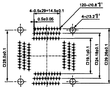
IC51-1204-1652 (120 Pins)
