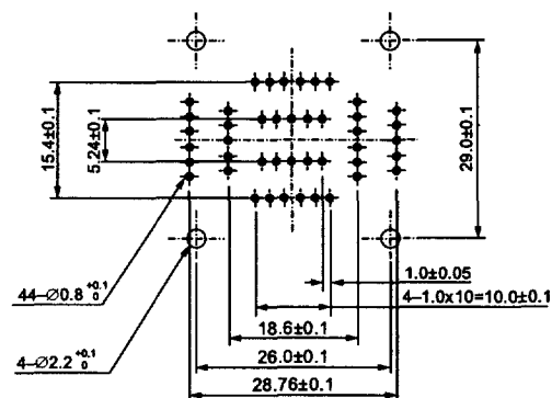
IC51-0444-615 (44 Pins)
