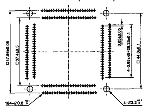
IC51-1844-1148-1 (184 Pins)
