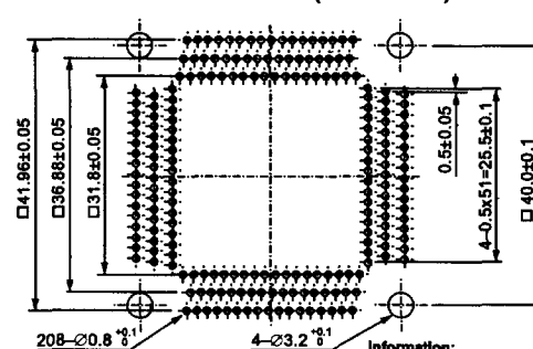
IC51-2084-1052-* 2) (208 Pins)
