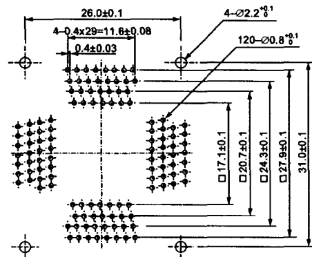
IC51-1204-1812 (120 Pins)
