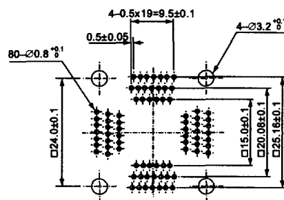
IC51-0804-711 (80 Pins)
