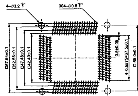
IC51-3044-1471-5 (304 Pins)
