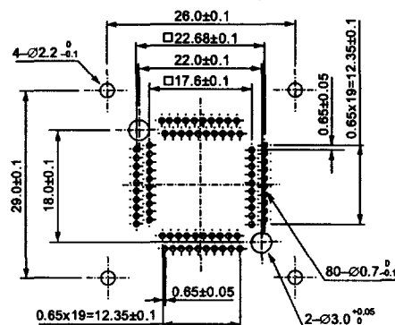
IC51-0804-956-2 (80 Pins)
