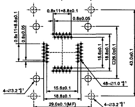
IC51-0484-081 (48 Pins)
